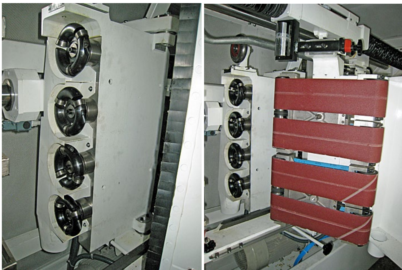
主軸ベルカッター \phi 35 \times 4 段 と サンディング装置 \phi 60 \times 4 連
